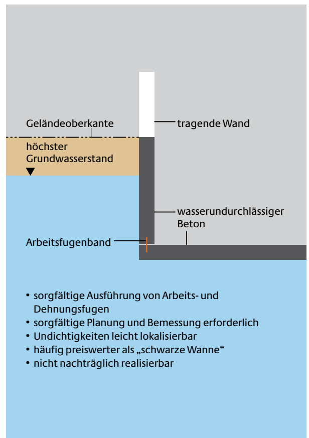
„Weiße Wanne“
